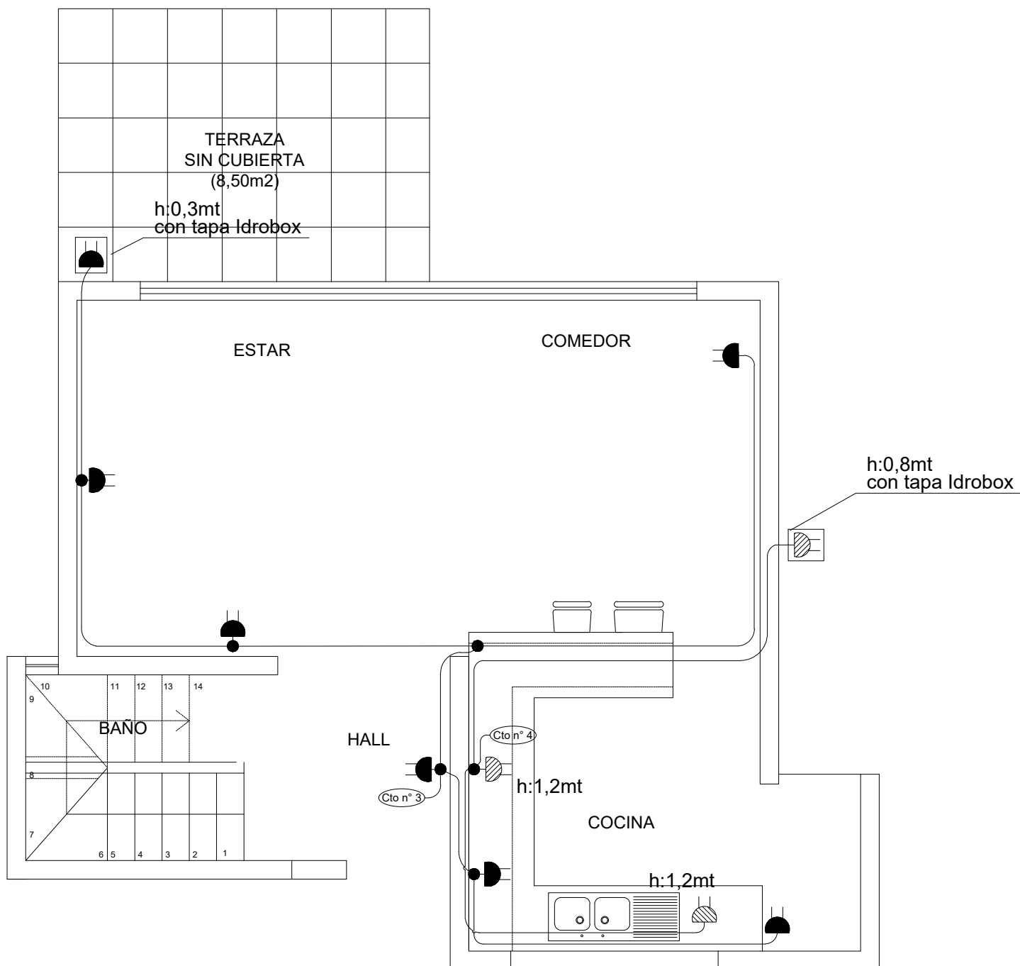
PLANTA ENCHUFES 1° PISO CASA TIPO AIRE
